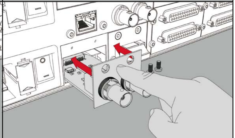
D Insert Madi-Module
